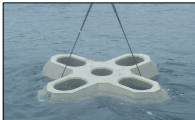
基礎の流出防止対策 (被覆ブロック据付)
