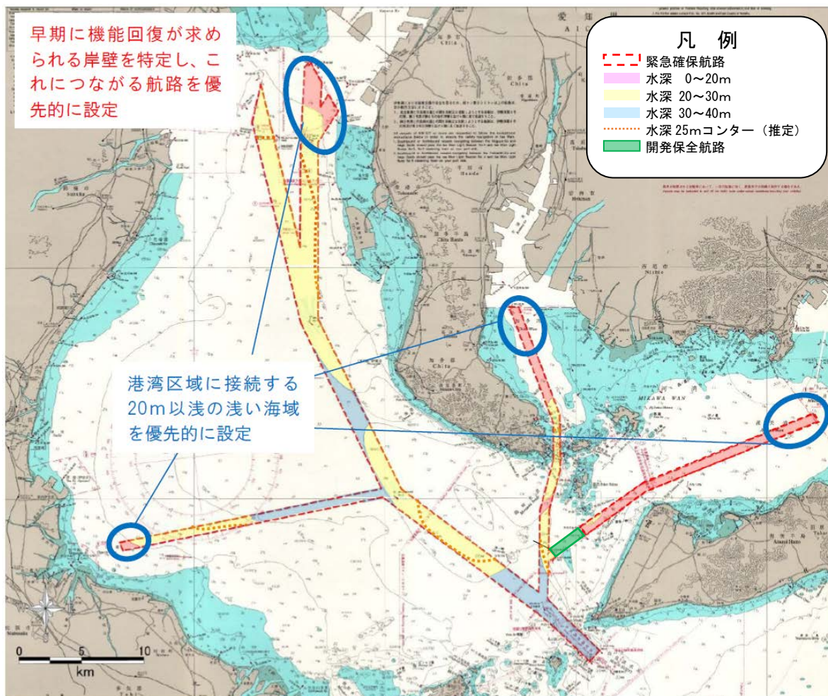
図 11 伊勢湾緊急確保航路において深浅測量（事前）を優先すべき海域
