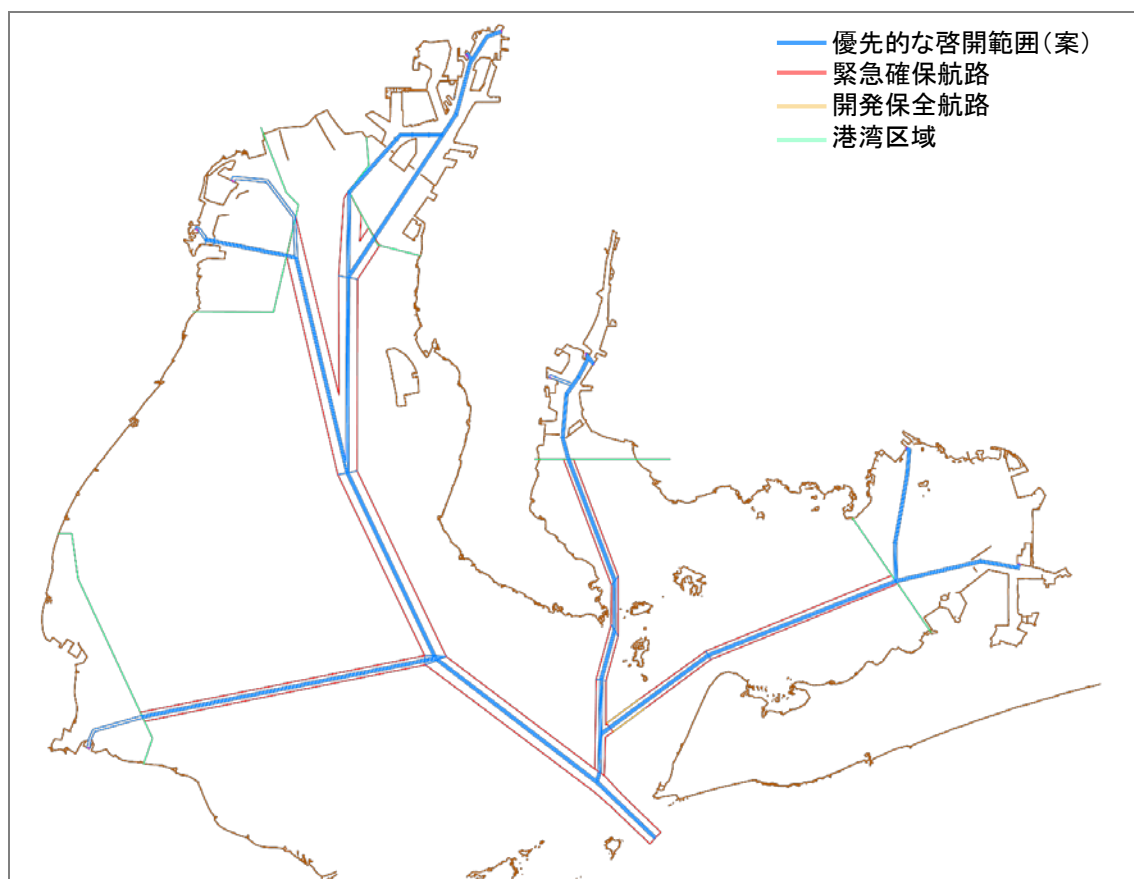
図 5 緊急物資輸送の暫定ルート
