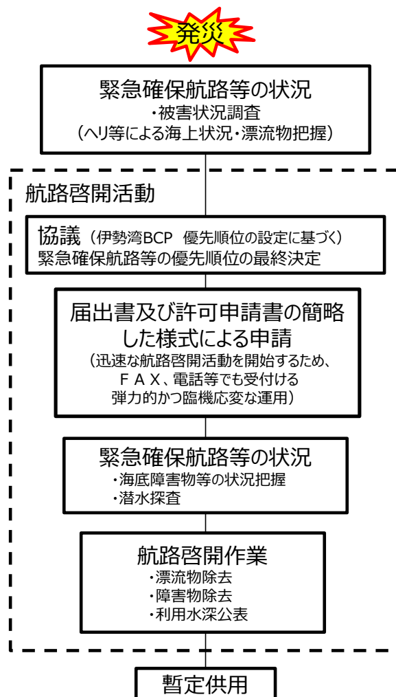
図 10 航路啓開の手順
