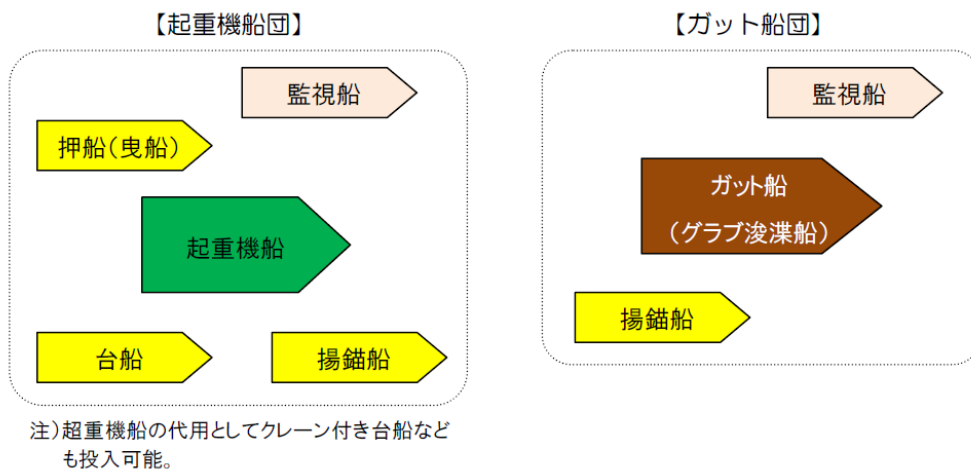
図 17 揚収作業において想定される船団構成
