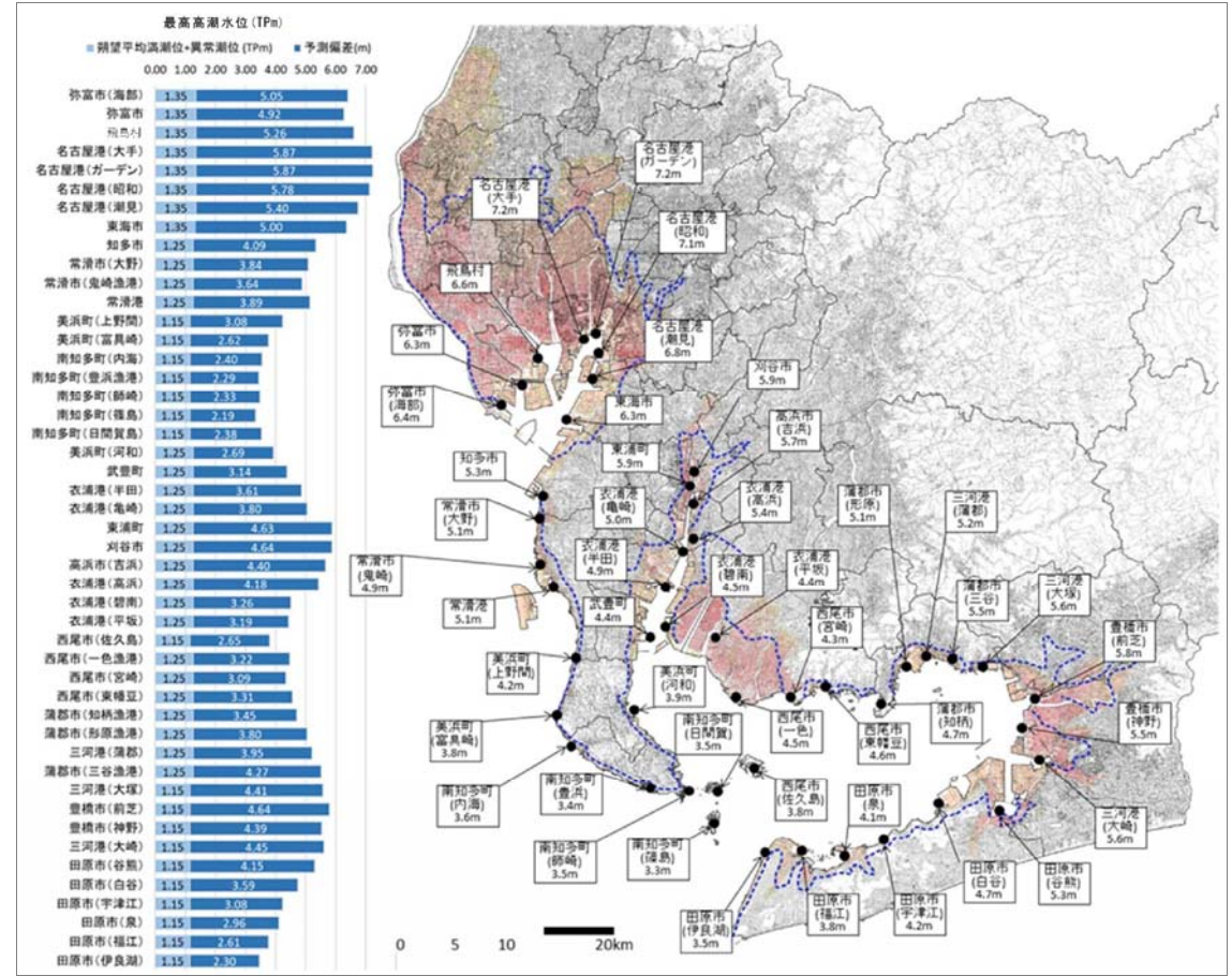
図 5 伊勢湾沿岸の高潮浸水想定（愛知県区間）
