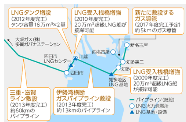
図 52 伊勢湾内の主な LNG 設備
