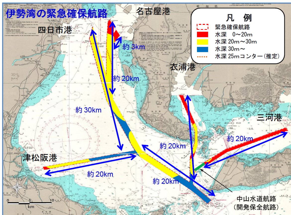
図 2 伊勢湾の緊急確保航路
