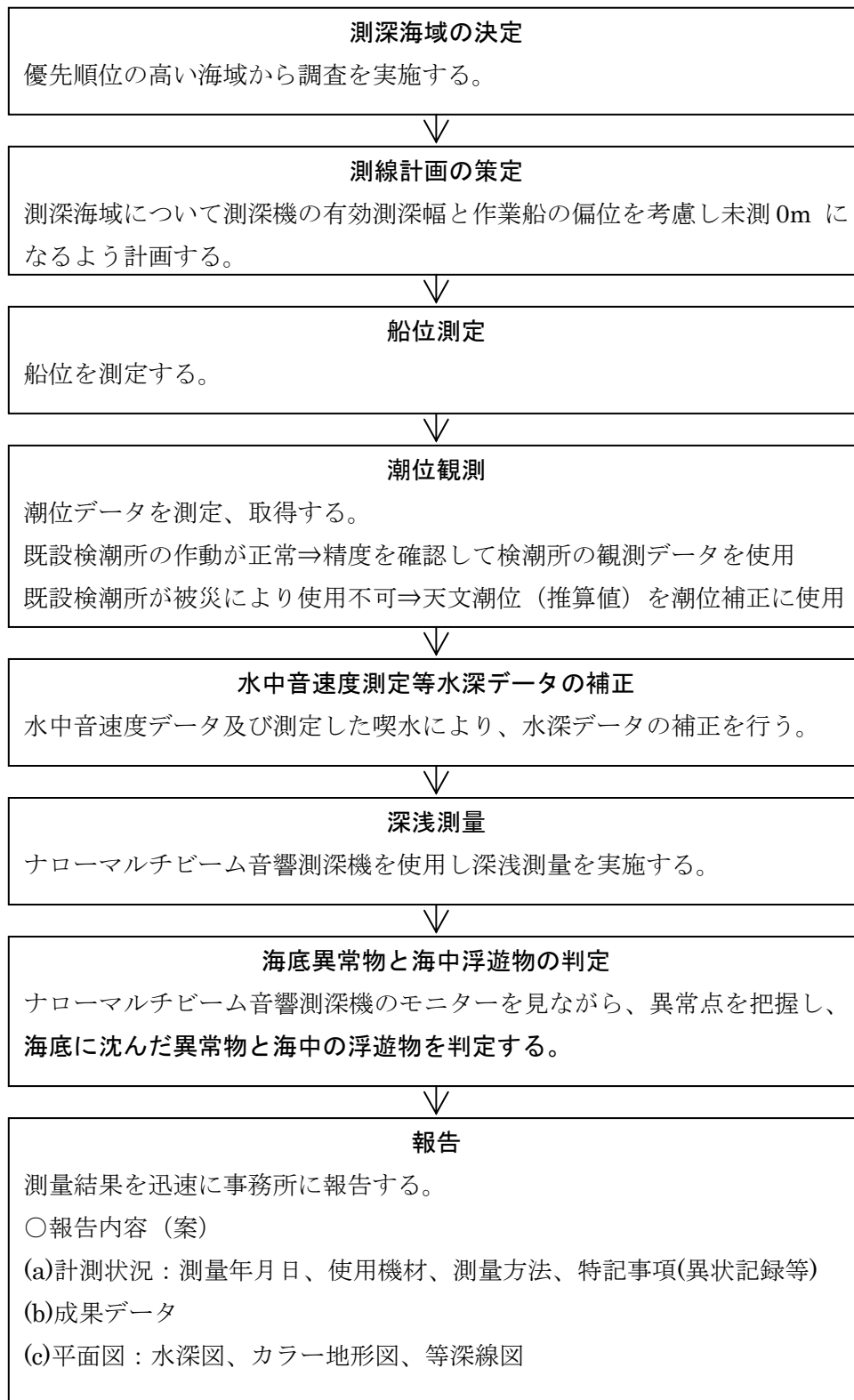
図 17 深浅測量（事前）の手順
