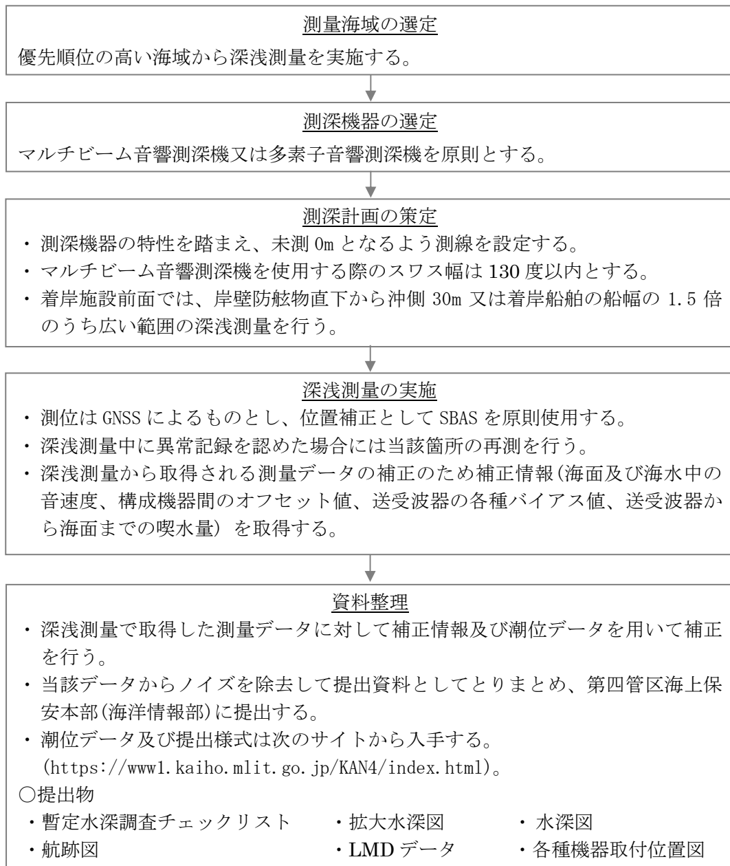
図 13 深浅測量（事後）の手順
