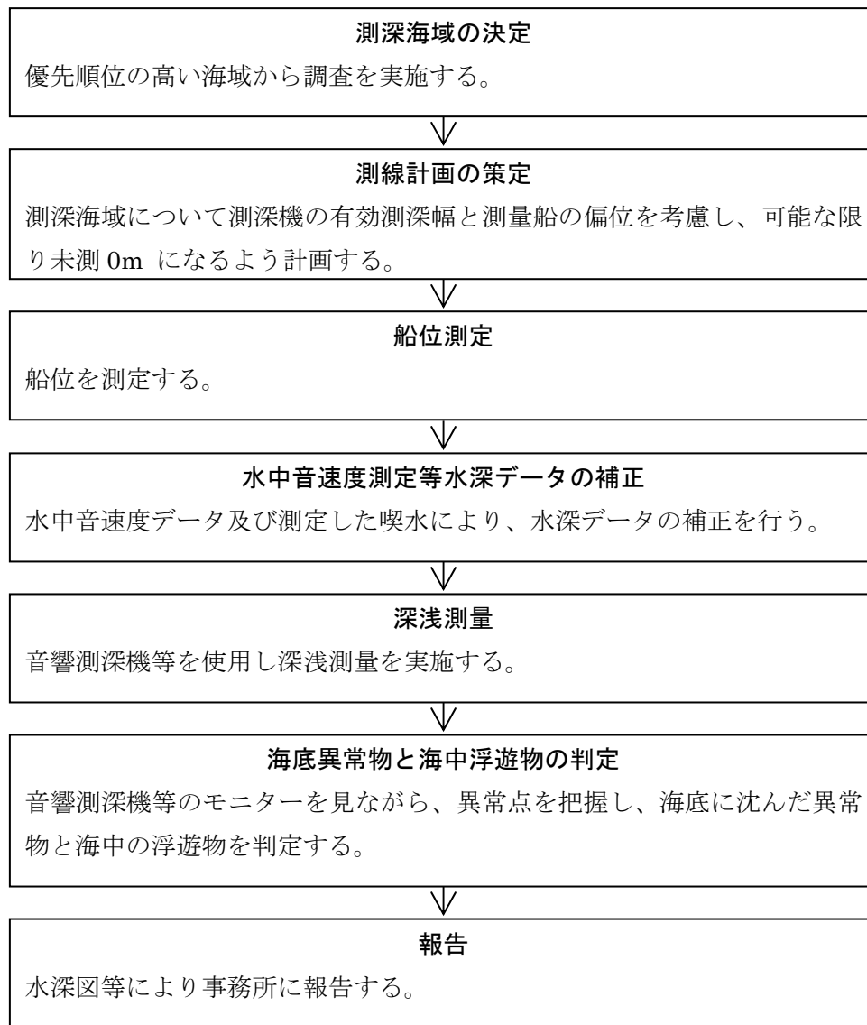
図 12 深浅測量（事前）の手順
