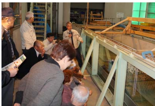
高潮防波堤断面模型の津波越波実験の様子
