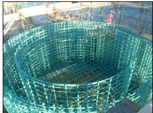
【②(鋼管矢板基礎)鉄筋組立状況】
